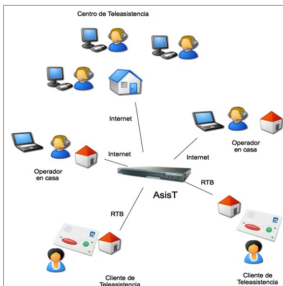
Esquema del sistema con centralita AsisT.
